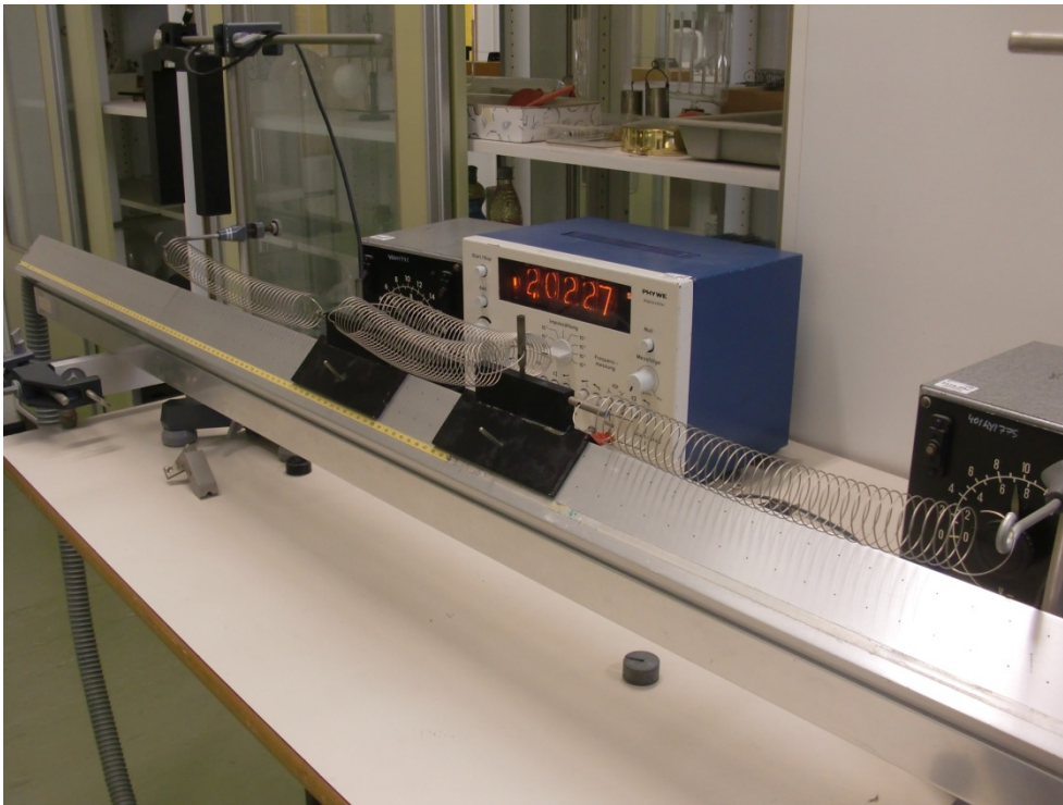
Abbildung 3 Versuchsanordnung
