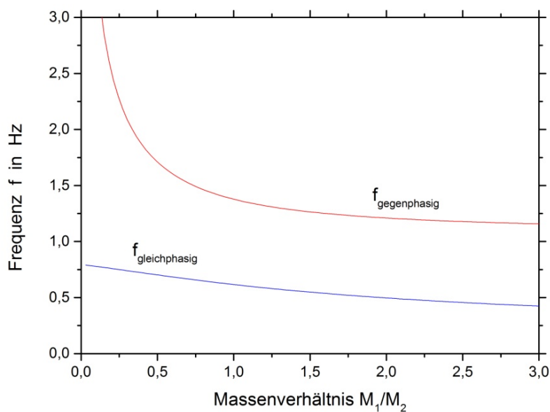
Abbildung 2 Frequenzen der Normalschwingungen der gekoppelten Pendel in Abbildung 1 , als Funktion des Massenverhältnisses M_2/M_1 . Theoretische Berechnung für D' = 3 \text{ N/m} , D = 6 \text{ N/m} und M_1 = 0,2 \text{ kg} . Rot: Gegenphasige Bewegung - Plus-Zeichen in Gleichung (4), Blau: Gleichphasige Bewegung - Minus-Zeichen in Gleichung (4)
