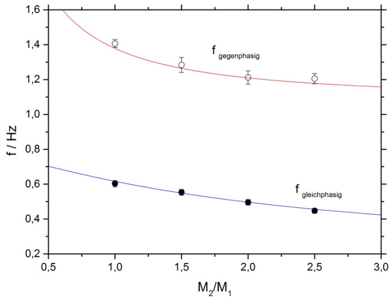
Abbildung 4 Messpunkte für D' = 3 \text{ N/m} , D = 6 \text{ N/m} und M_1 = 0,2 \text{ kg} und die nach Gleichung (4) berechneten theoretischen Kurven. Wie in Abbildung 3 gilt: Rot entspricht der gegenphasigen Bewegung, also dem Plus-Zeichen in Gleichung (4), Blau der gleichphasigen Bewegung und dem Minus-Zeichen in Gleichung (4)
